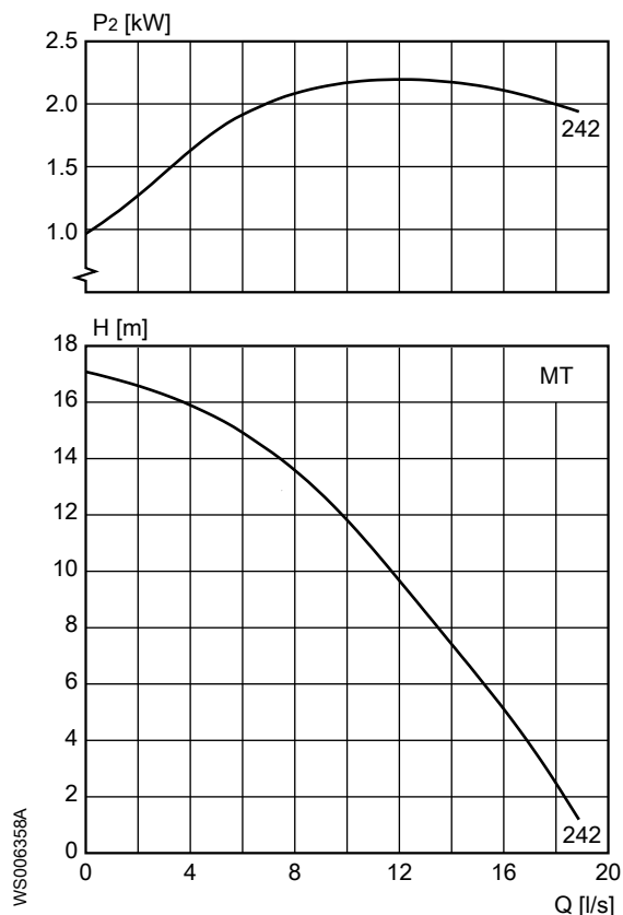
Afbeelding 10: 60 Hz
