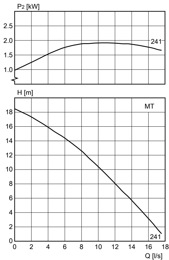
Afbeelding 9: 50 Hz
