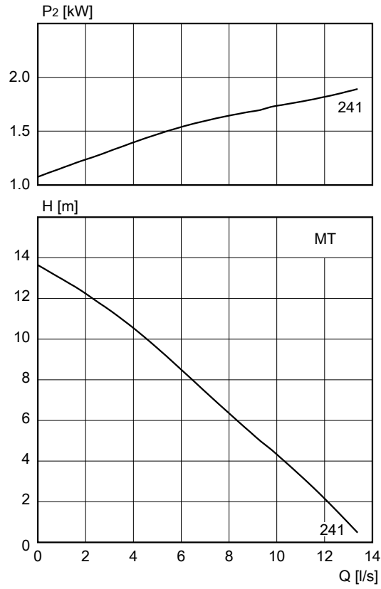
Afbeelding 7: 50 Hz
