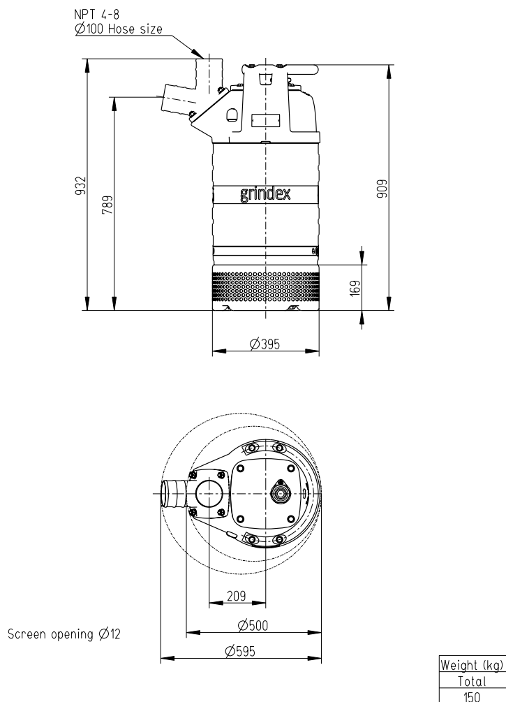
Afbeelding 12: MSHA-uitvoering, H
