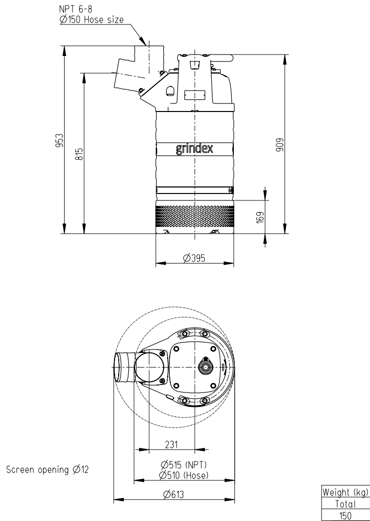
Afbeelding 11: MSHA-uitvoering
